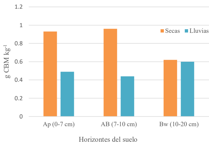
Figura 3. Carbono de biomasa microbiana en el sistema A-1. Figure 3. Microbial biomass carbon in system A-1.
