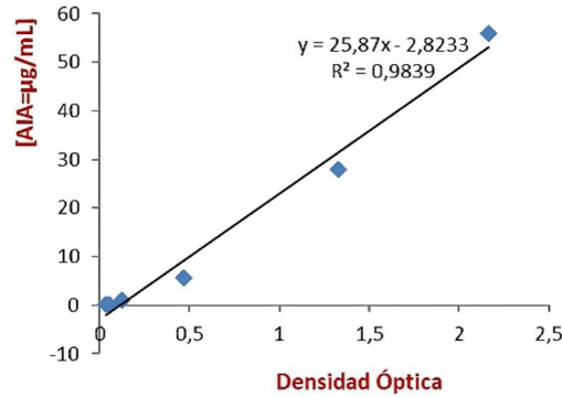
Figura 2. Determinación de la curva estándar de Ácido Indolacético Figure 2. Determination of the Indol Acetic Acid standard curve.
