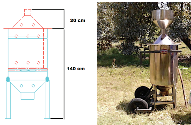
Figura 2. Equipo (PAM) construido en acero inoxidable con volumen útil de 0.05 m 3 .
